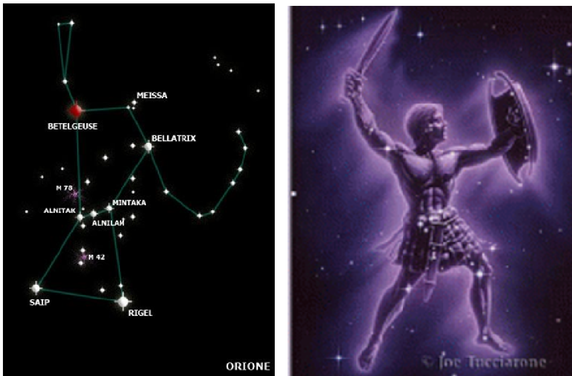
FIGURE 27. CONSTELLATION D'ORION
